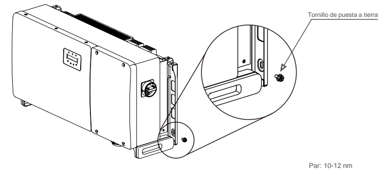
Figura 3.17 Cable fijo
